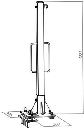
Рис. 1 – Габаритные размеры
